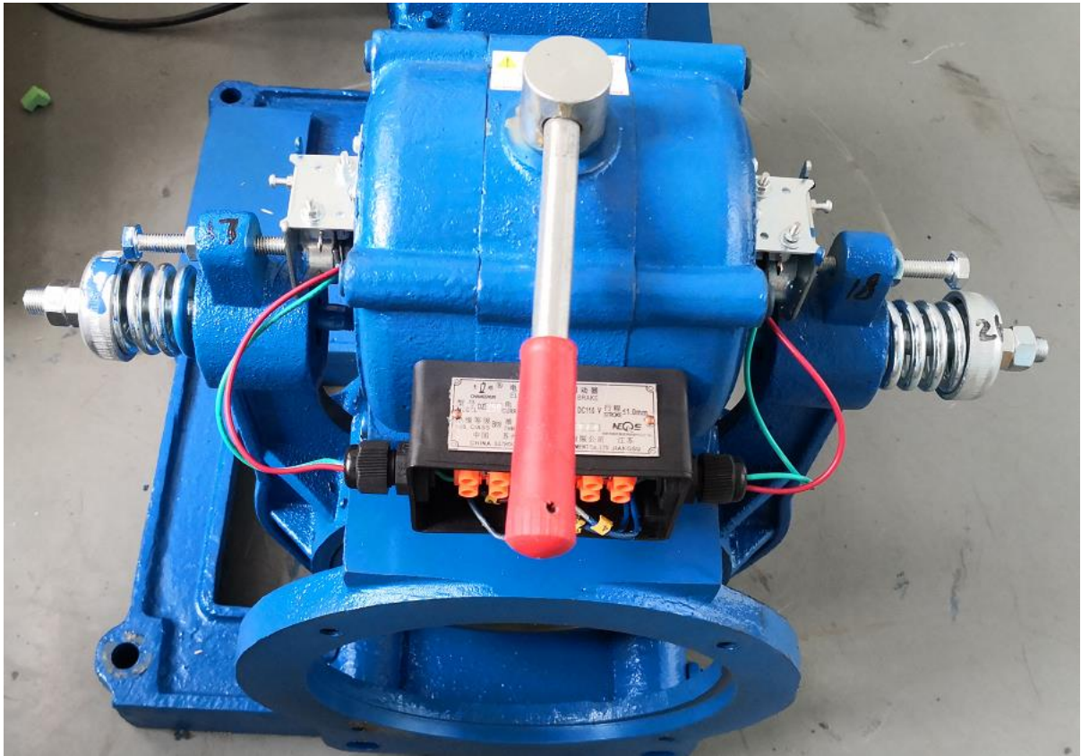
DZ250 型鼓式制动器
