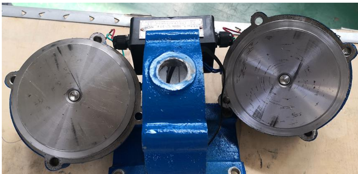
600 次手动松闸试验后的铁芯端面
